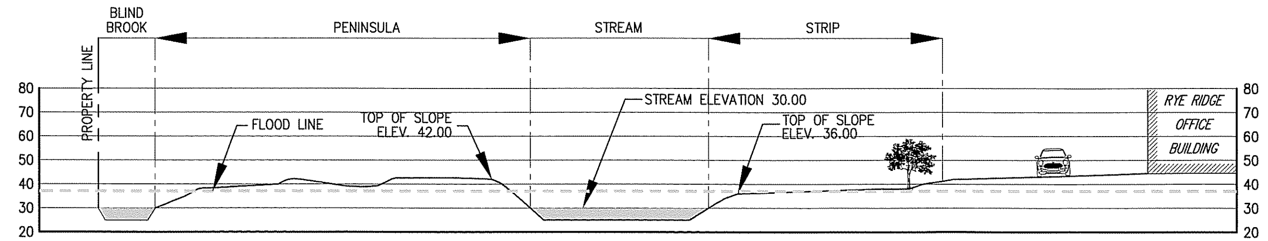
SECTION A-A SCALE: H: 1"=40' V: 1"=40'
